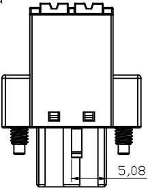
2P外壳抓扣 排列示意
